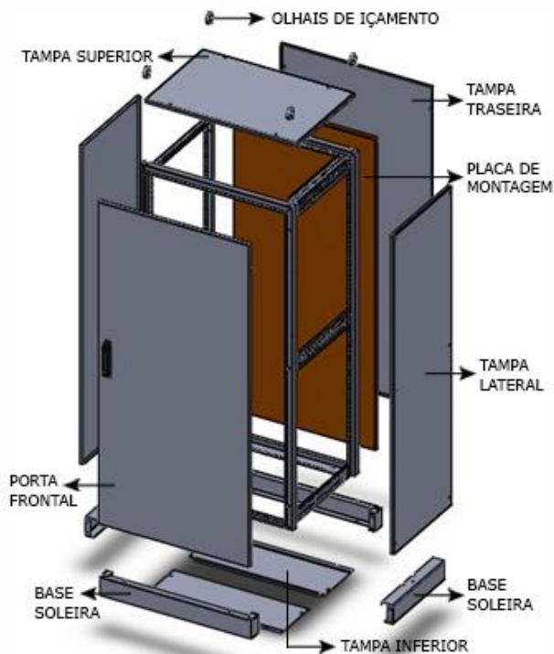
Porta frontal única Painéis de Largura 600 e 800mm
